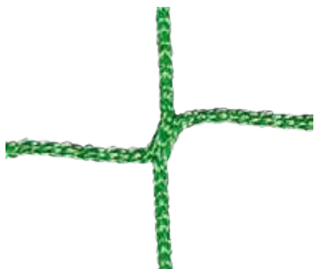
Č. 209 zelený, bezuzlový vysokopevnostní polypropylen, \varnothing cca 3 mm
