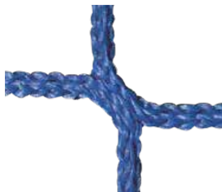
Č. 212 modrý, bezuzlový vysokopevnostní polypropylen, ø cca 5 mm
